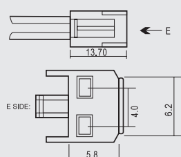
JST-Stecker
