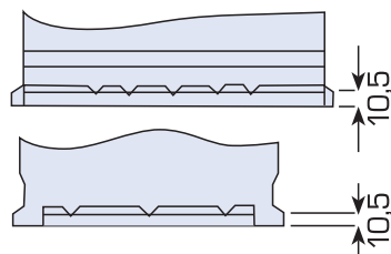
Bodenleiste B13
