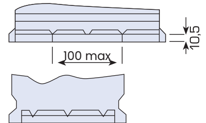
Bodenleiste B3
