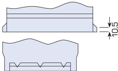
Bodenleiste B11
